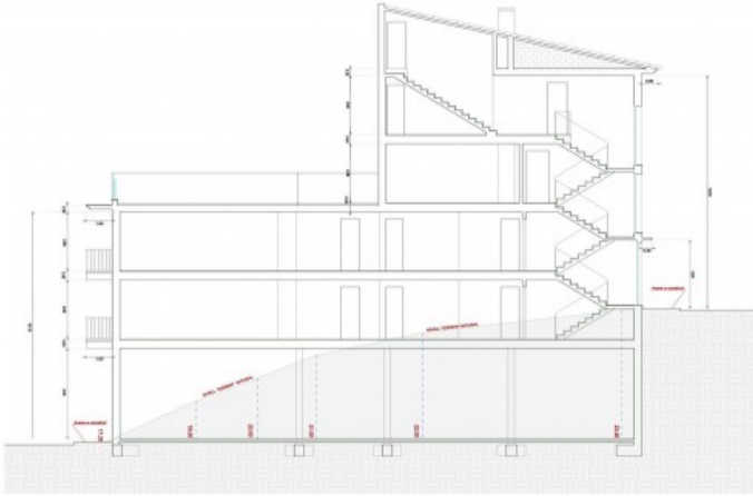
SECCIÓ A-A'
